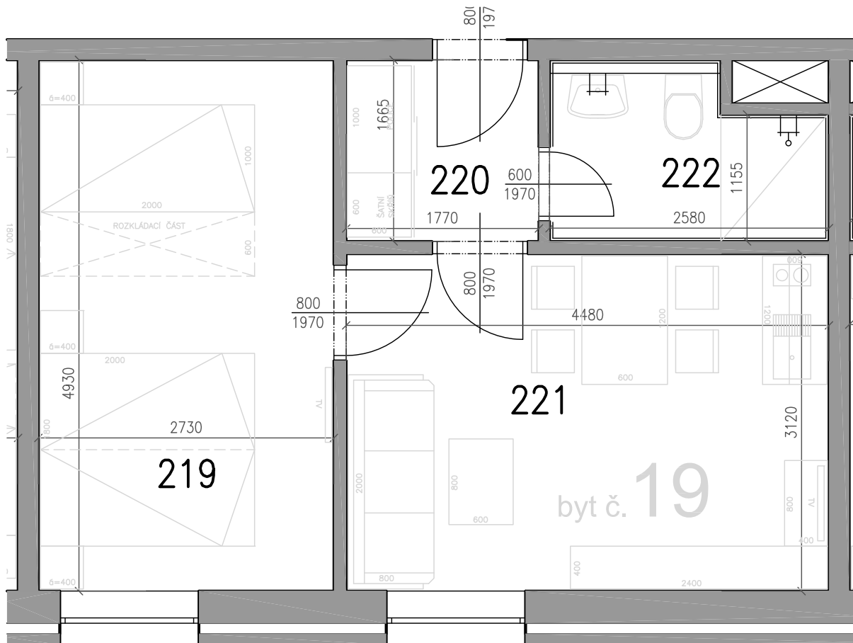
Půdorys bytu 1:50
