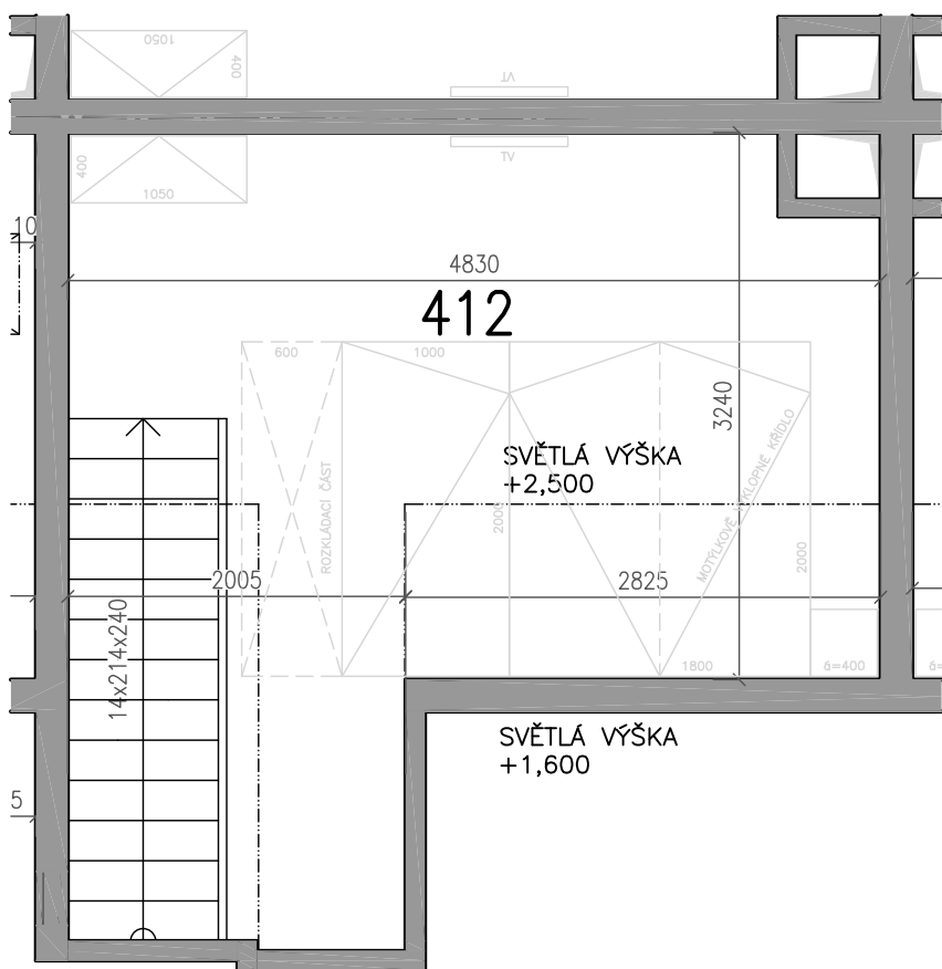
Půdorys bytu 1:50
