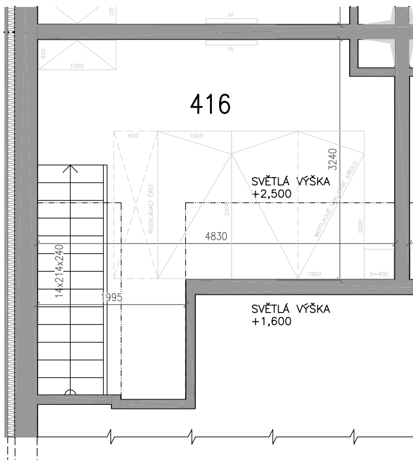
Půdorys bytu 1:50
