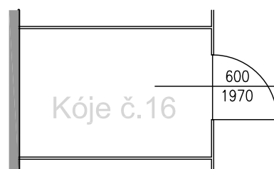
Půdorys sklepní kóje 1:50
