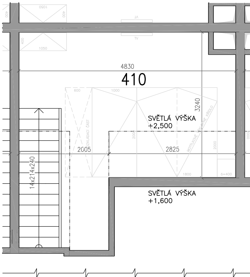
Půdorys bytu 1:50
