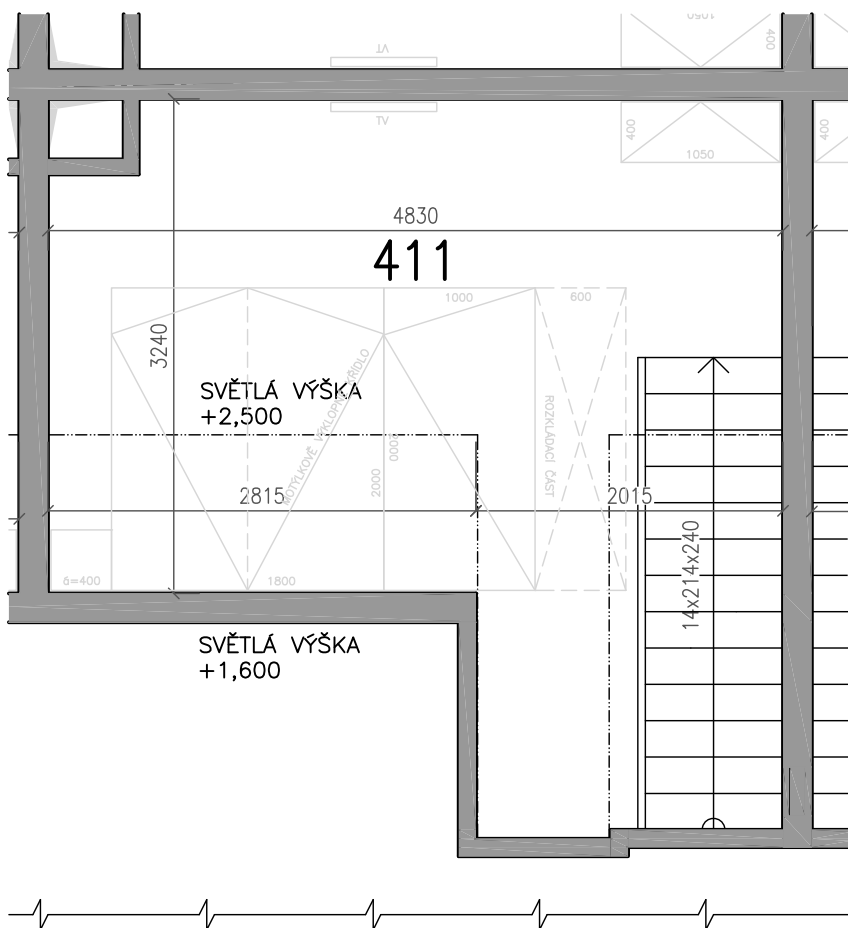
Půdorys bytu 1:50
